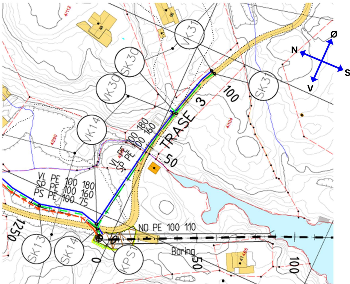
Fiesundveien mot øst (kum SK14 til kum SK31) - gravitasjonsledning for avløp
