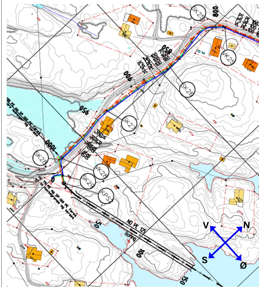
Åkvågvæien, Fiesundveien til Fiestrand (kum SK25 til kum SK29) - gravitasjonsledning for avløp
